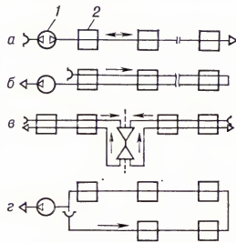
Рис. 4. Схемы соединения станций пневматической почты: а — линейная однострубная; б — линейная двухтрубная; в — радиальная; г — кольцевая; 1 — воздуходувка; 2 — станция.
